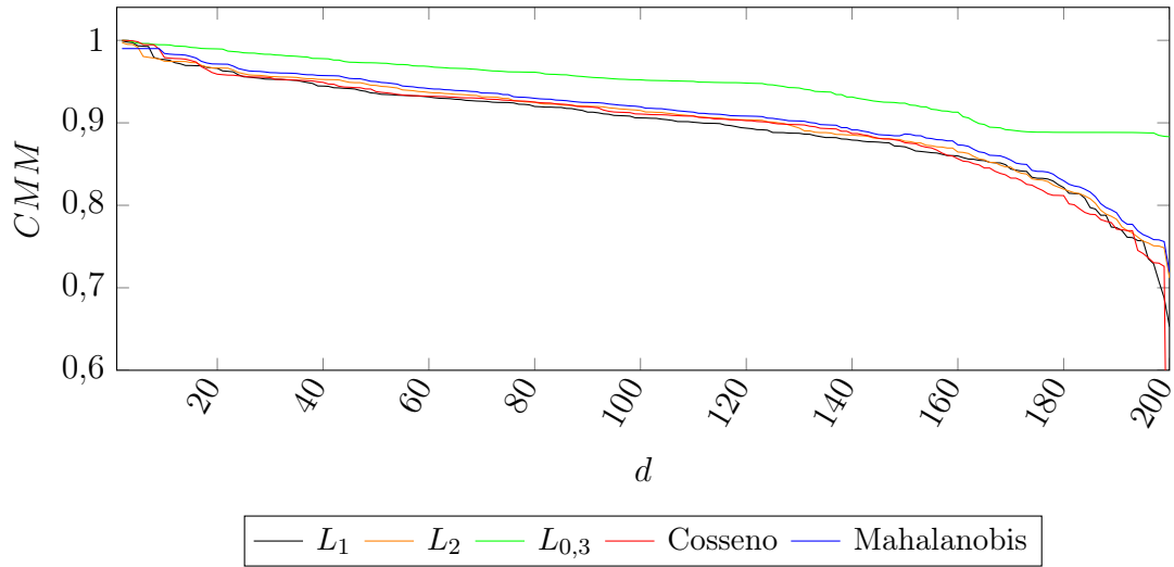
Figura 5.12: CMM obtido pelo algoritmo SNCStream adotando diferentes métricas de distância ao variar a dimensionalidade d de um problema RBF.
