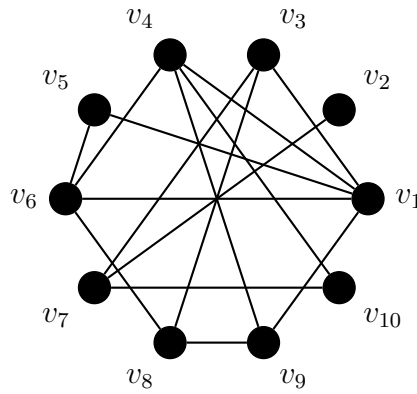
Figura 3.6: Exemplo de rede aleatória.
