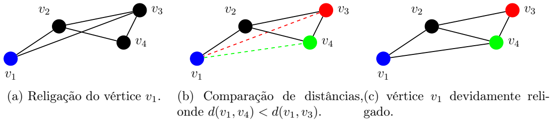
Figura 4.3: Exemplo de religação de v_1 , onde \deg(v_1) = 2 .
