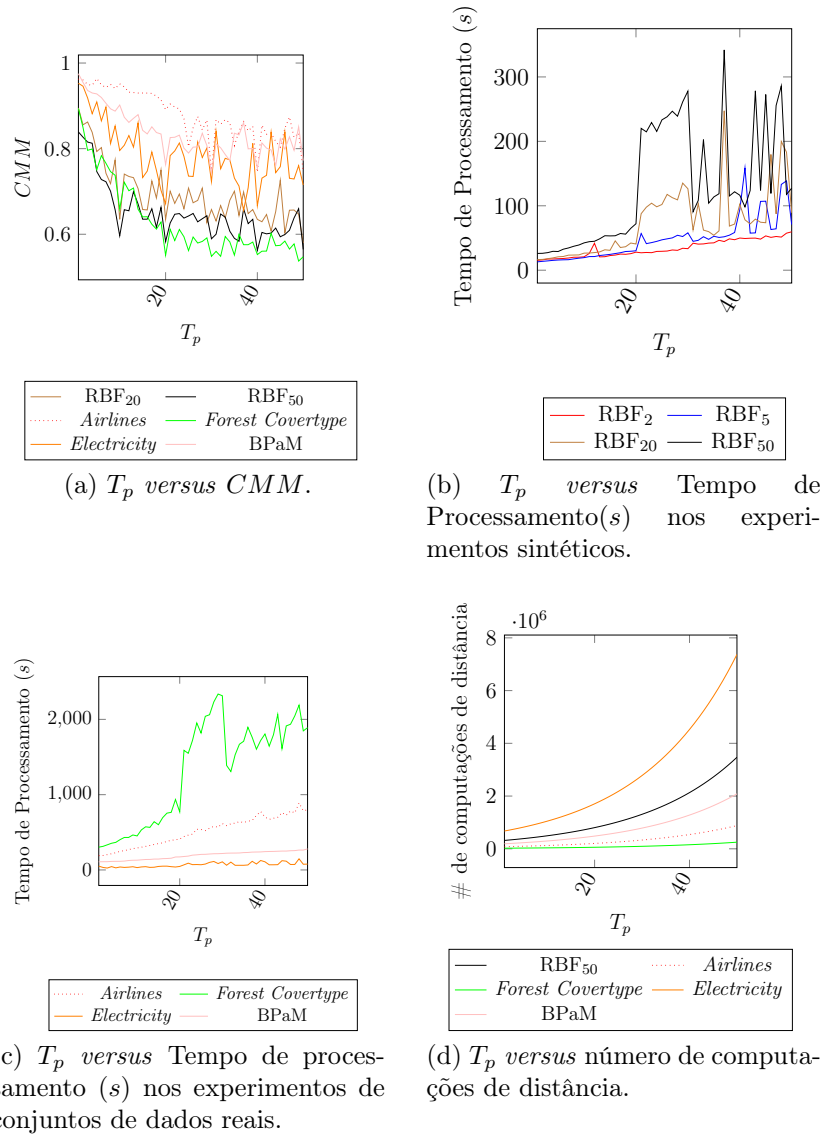
Figura 5.11: Resultados obtidos ao variar T_p .
