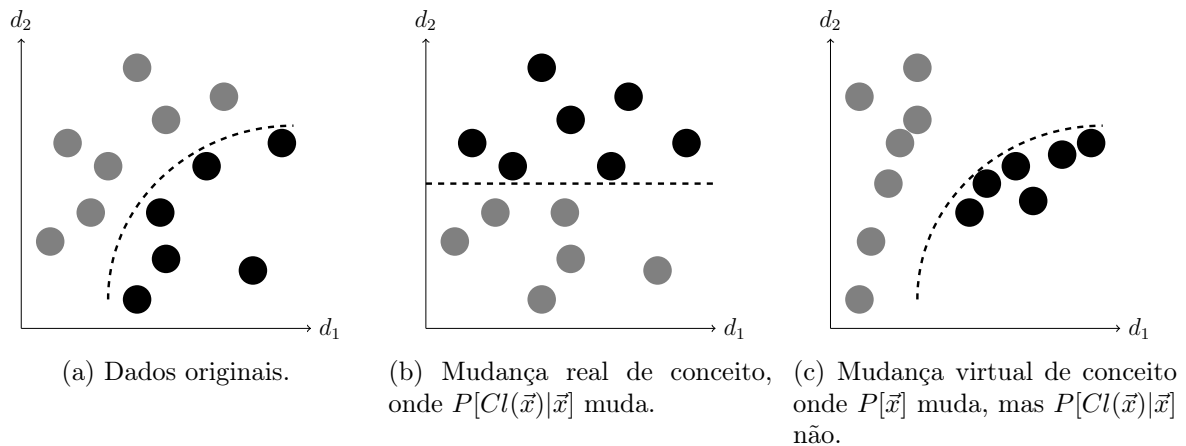
Figura 2.1: Tipos de mudança de conceito: círculos representam instâncias, níveis de cinza diferentes representam classes diferentes e a linha tracejada define o limiar de separação inter-classes.
